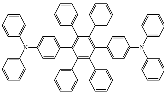
TATT
