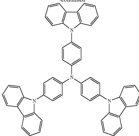
TCTA
