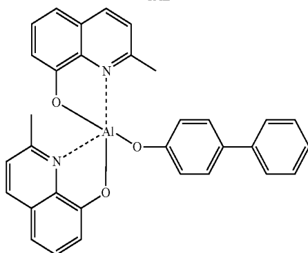
BAlq
